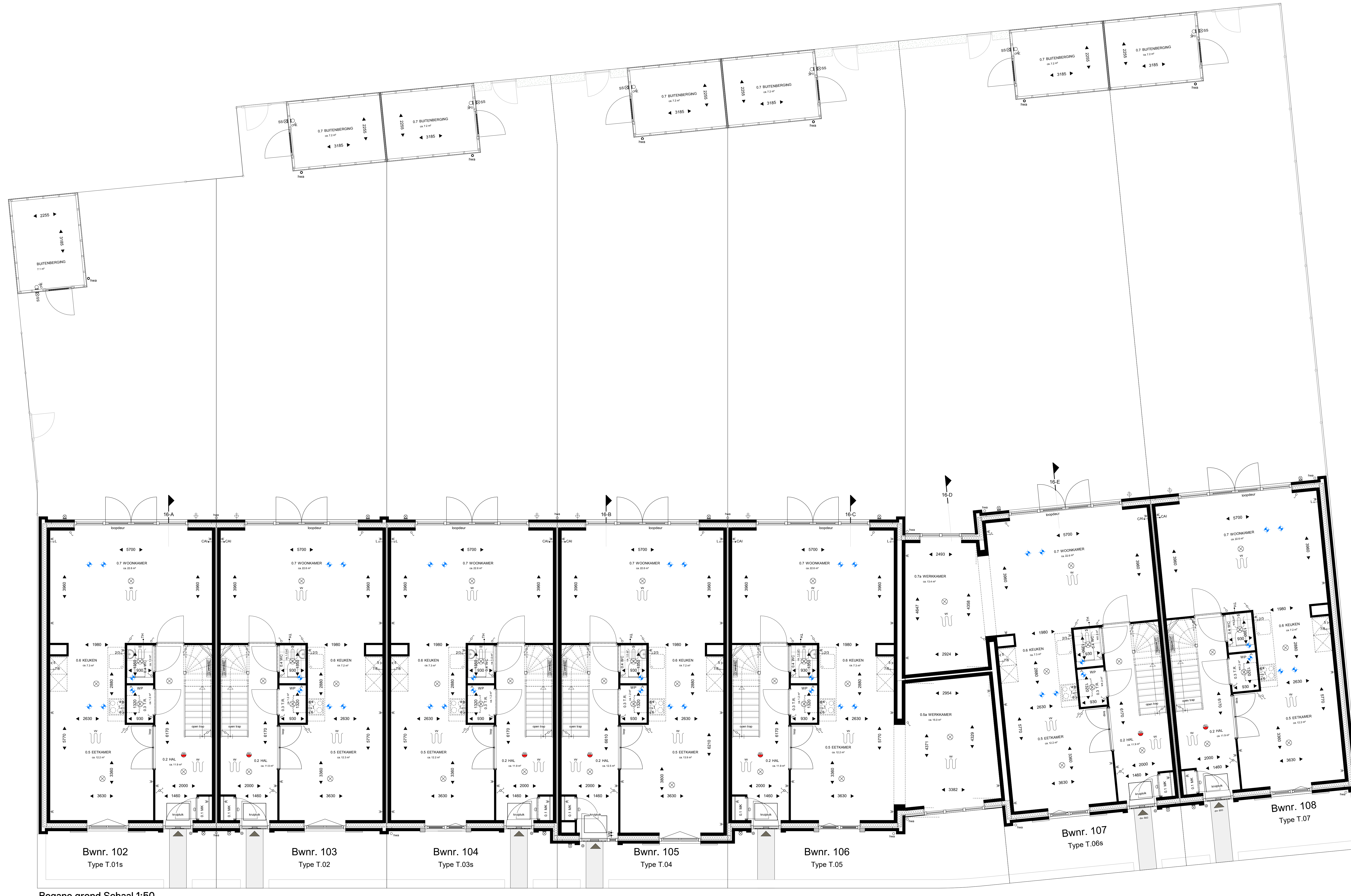
Begane grond Schaal 1:50
